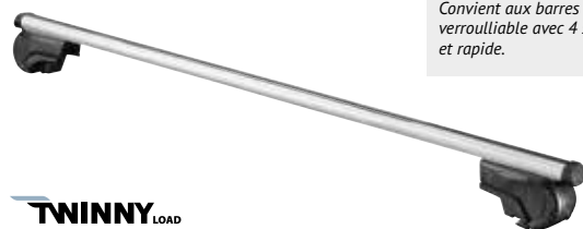
Dakdragerset "Fly Bar" 124cm. Max. belastbaar: 100kg / Porte charges de toit "Fly bar" 124cm. Max. belastbaar: 100kg
