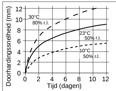
Schema 1: Uithardingstijd voor Sikaflex®260 N
