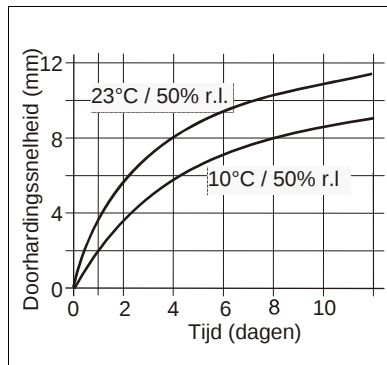
Schema 1: Doorhardingssnelheid voor Sikaflex®-256
